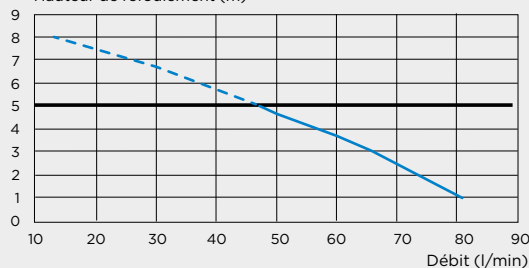
Hauteur de refoulement (m)
